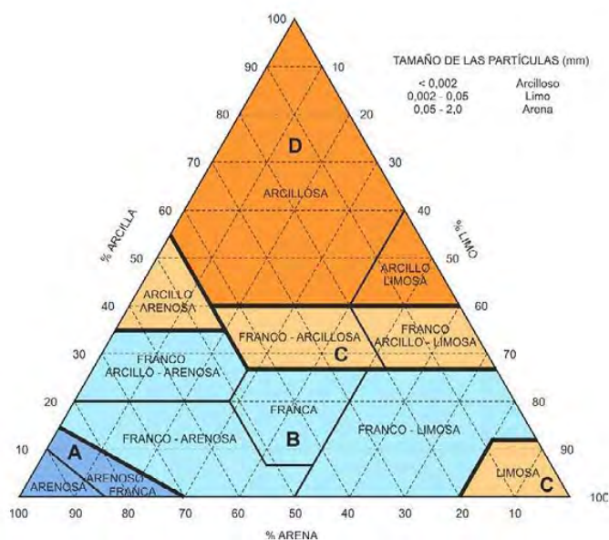
Diagrama triangular para determinación de la textura en materiales tipos suelo
