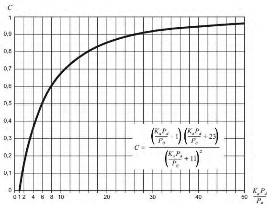
Determinación del coeficiente de escorrentía
